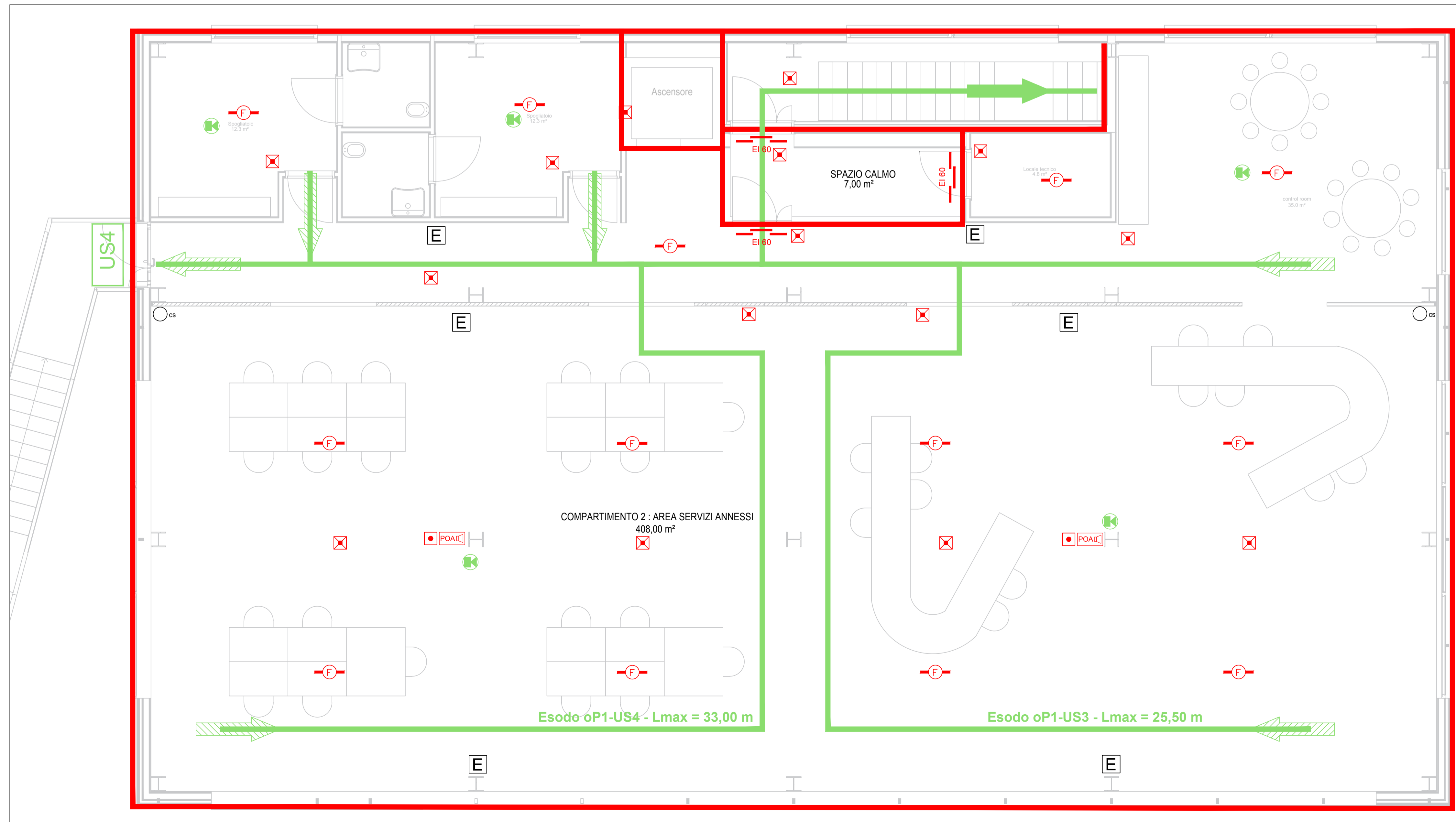
PIANTA PIANO PRIMO - SCALA 1:50
